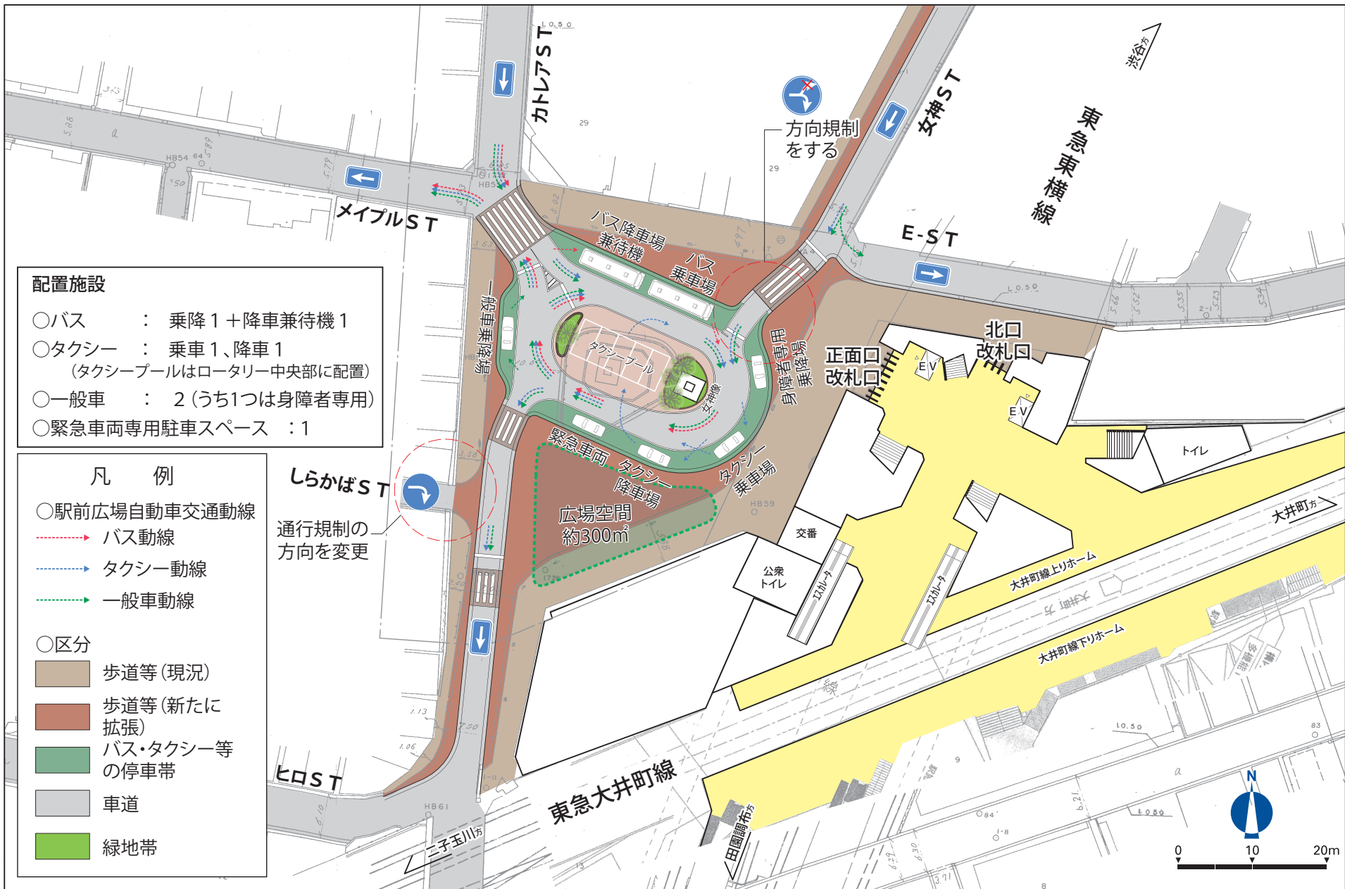
自由が丘駅前広場整備計画(案)
